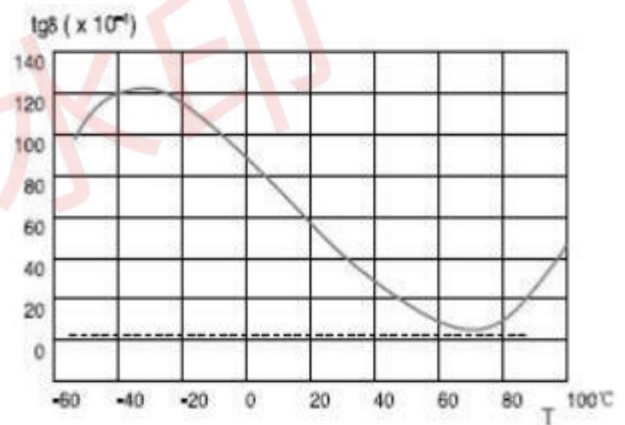
损耗角正切与温度曲线图
